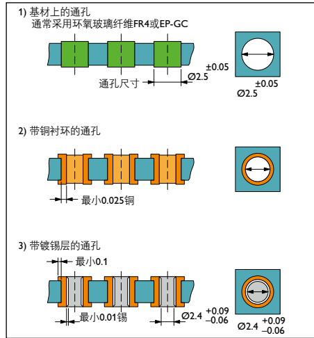
适配单排SDC 2.5的通孔内径 (单位：mm)
