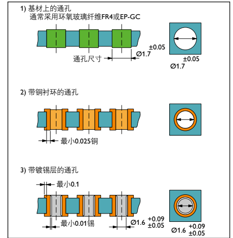
适配双排SDDC 1.5的通孔内径 (单位：mm)
