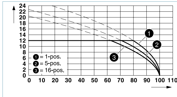
SDC 2,5系列
