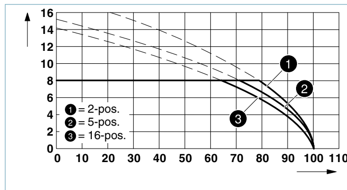
SDDC 1,5系列
